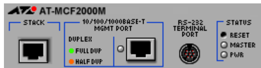
Management Module : 10/100/1000BASE-T
